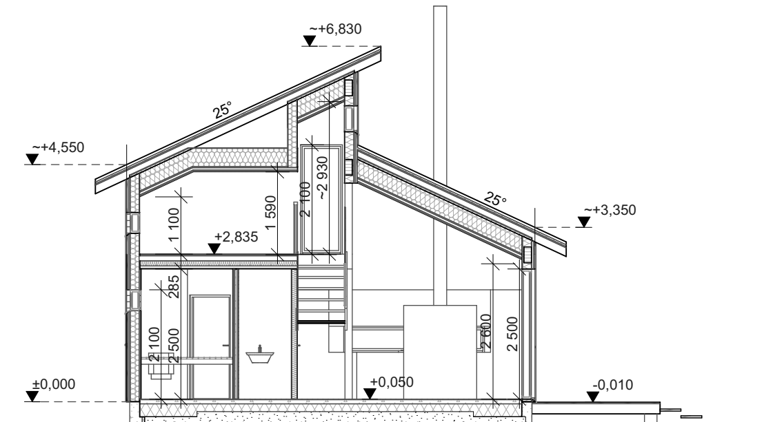
LEIKKAUS A-A
